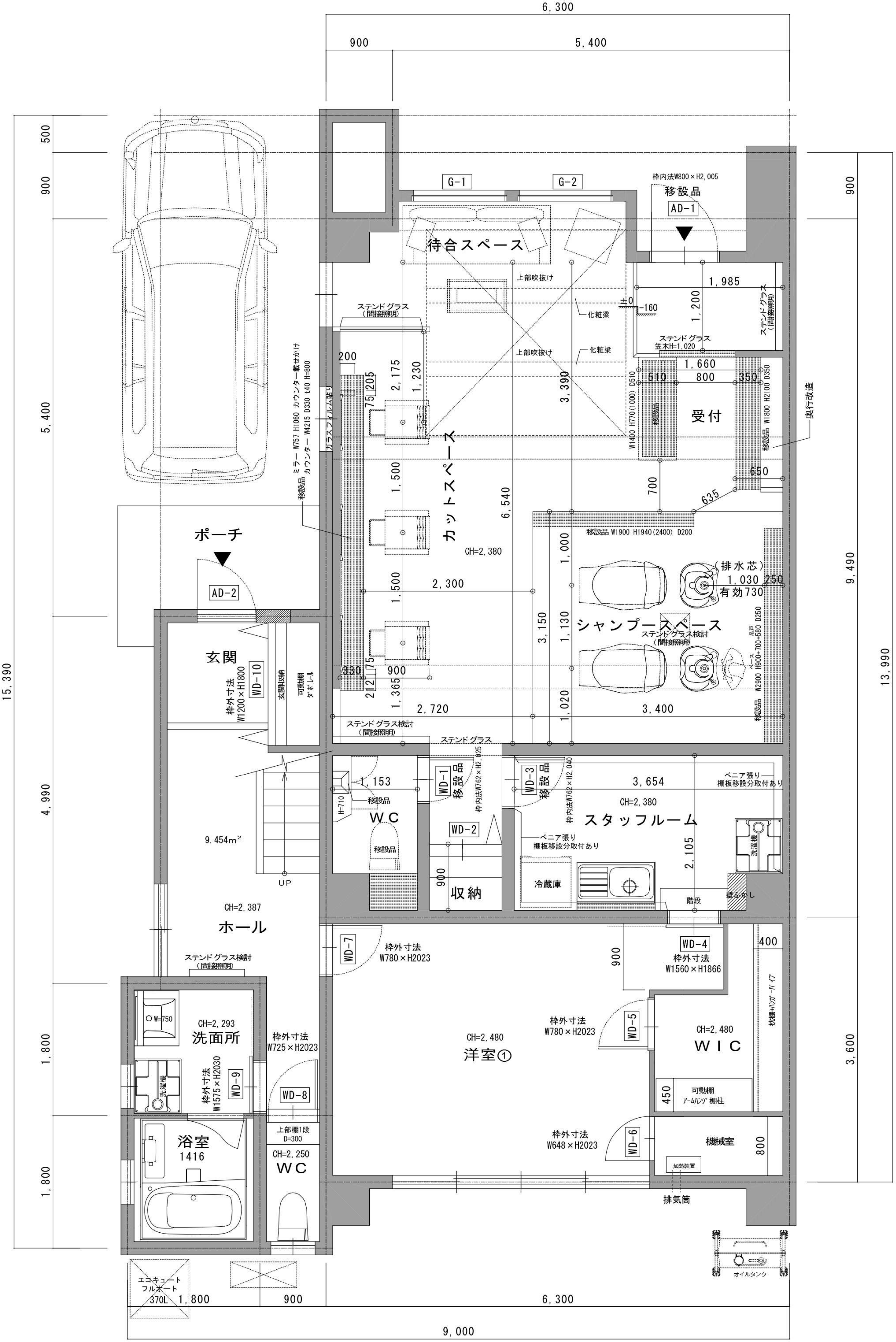
1階 平面図
