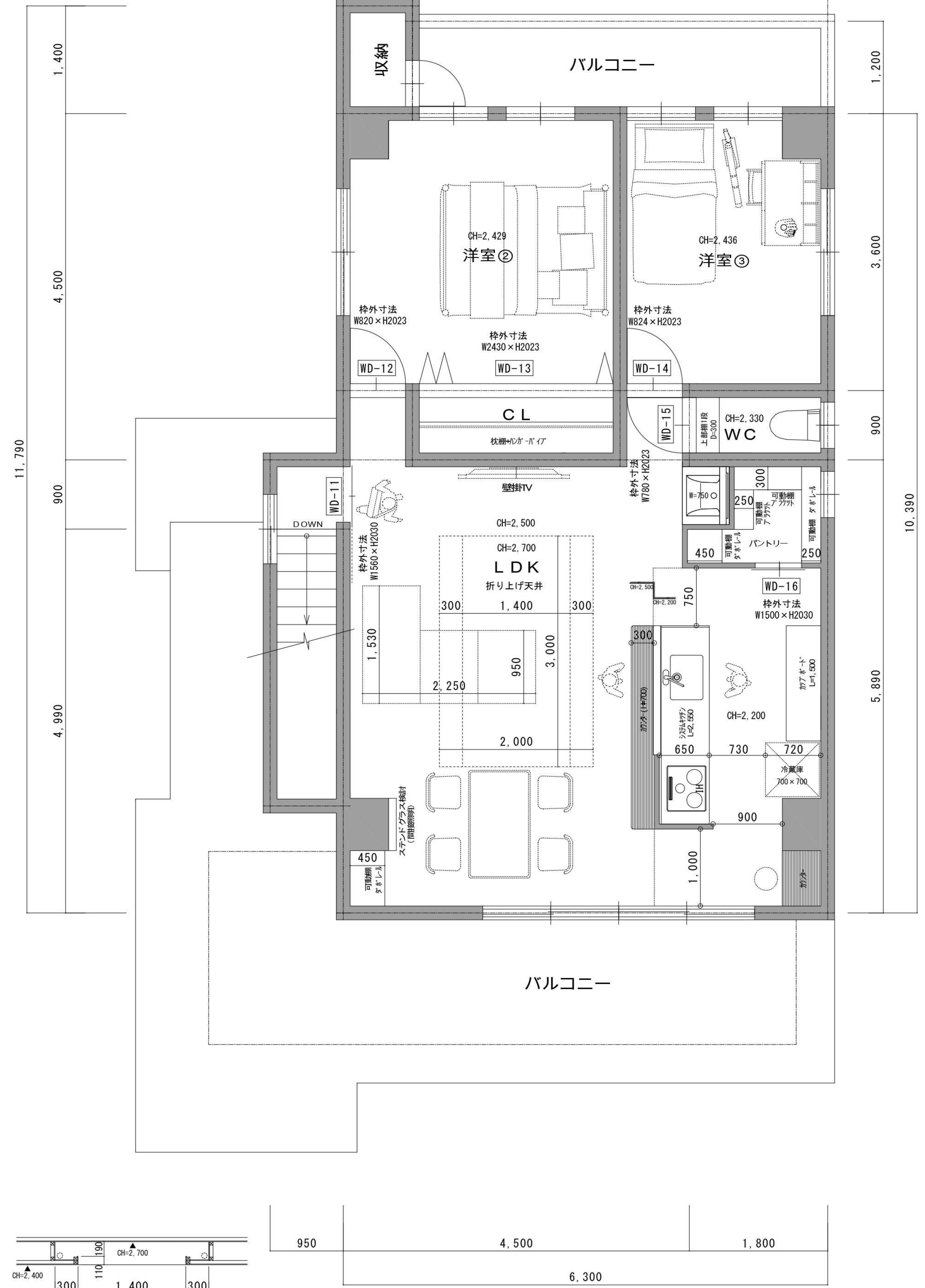
2階 平面図
