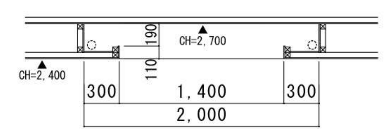
2F折り上げ天井詳細図
